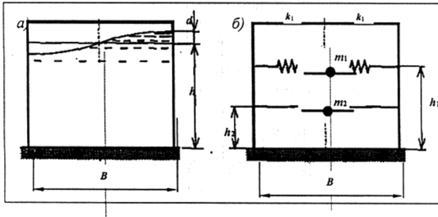
Рис.П.5.1. Моделирование резервуара с жидкостью:
